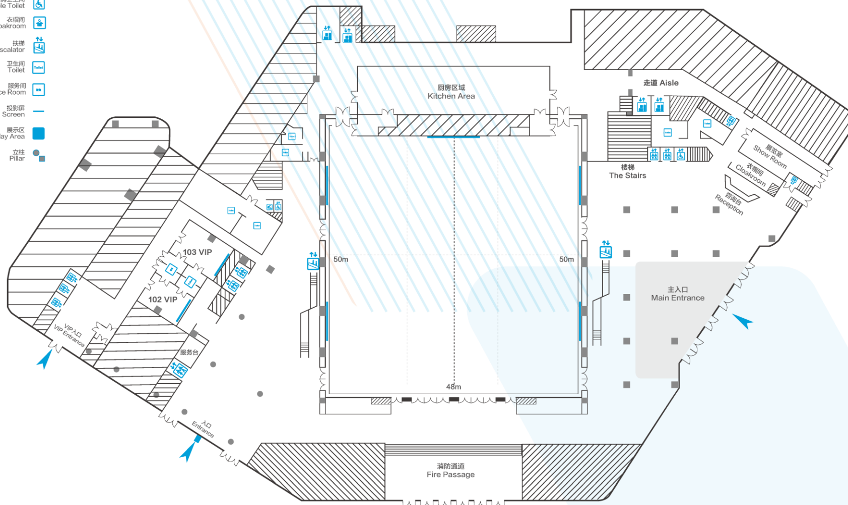
1 st FLOOR LAYOUT 一层平面图
